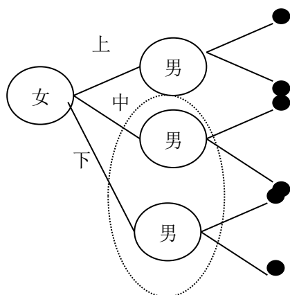
图 3-5 扩展式性别战 II
